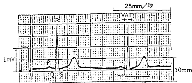
図4-16 心電図
