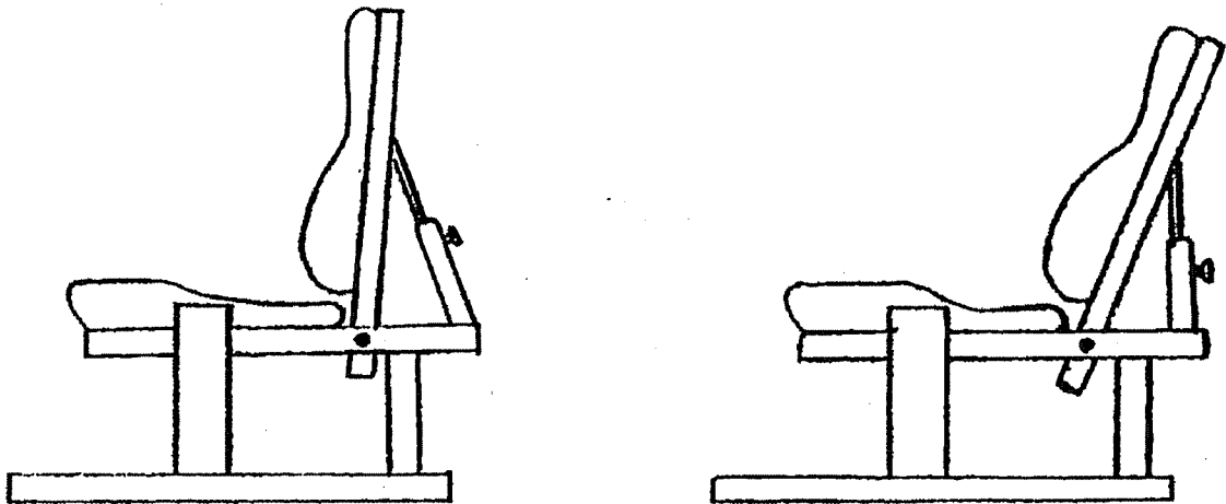
図－51 リクライニングの概念図
