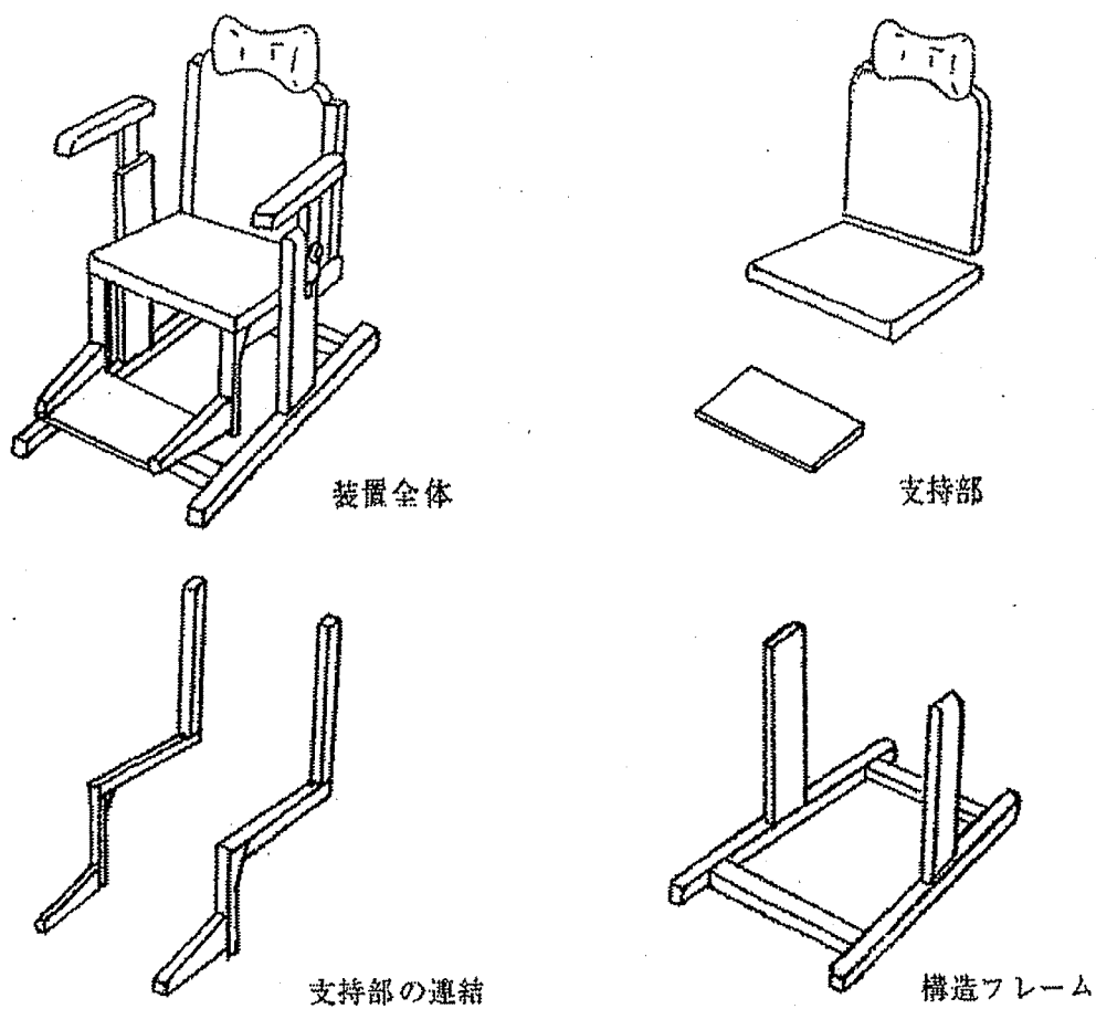
図－49 座位保持装置の構成概念図
