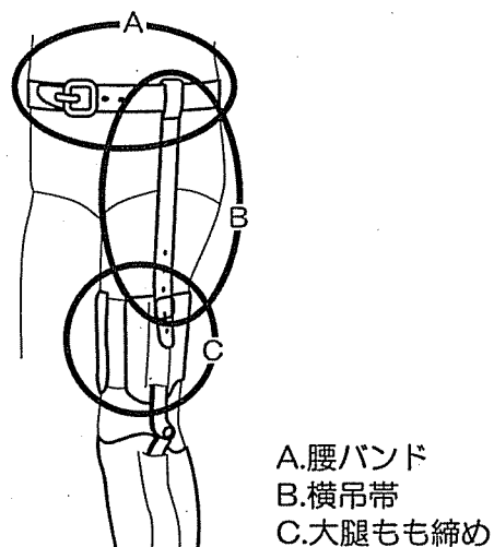
図-23 下腿義足懸垂用部品の区分
