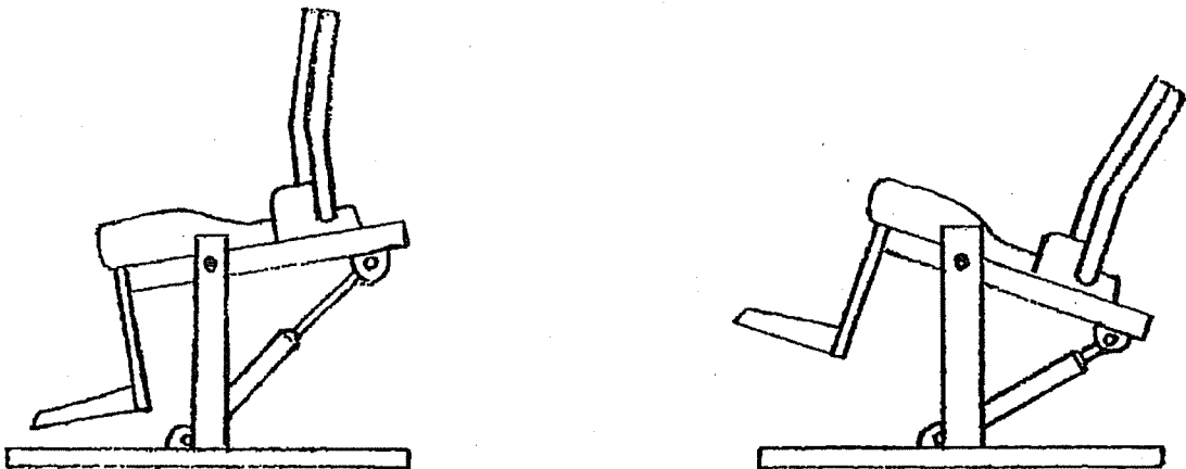
図－53 ティルト機構の概念図
