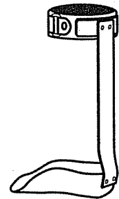
図-42 板ばね支柱の事例
