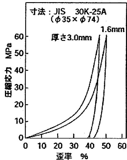
図 3.11 SUS 落入り膨張黒鉛シートの圧縮復元特性の例 8)
