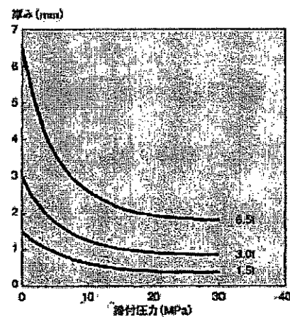
図 3.9 特殊加工 PTFE ガasket の締付面圧と厚さの関係の例 5)
