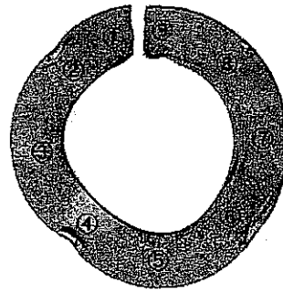
図 3.8 ブローアウトした充填材入り PTFE ガasket 4)
