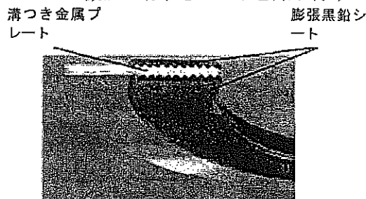
図 3.14 カンプロファイルガスケット 10)
