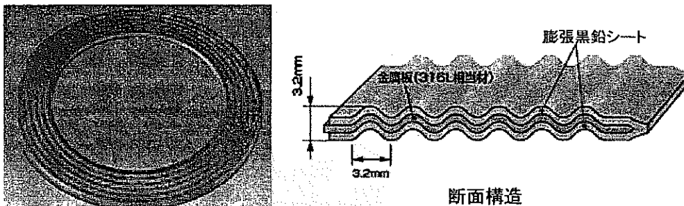
図 3.12 CMGC ガスケット 9)
