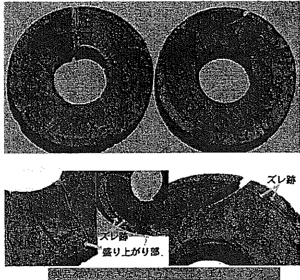
図 5.1 ガスケットの損傷
