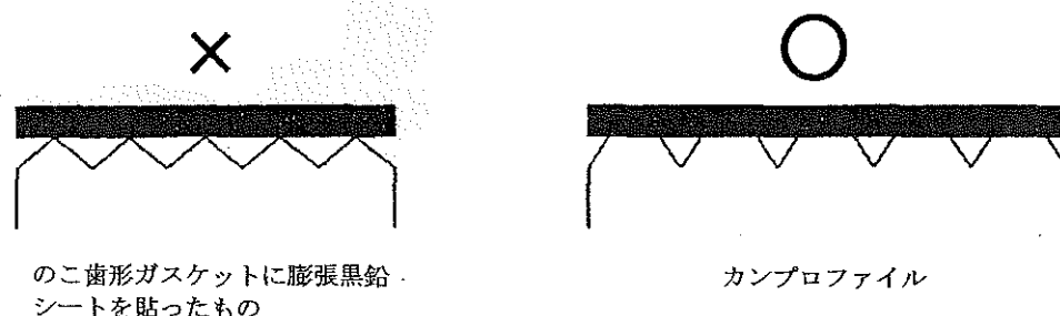
図 3.15 カンプロファイルと のこ歯形ガスケットに黒鉛シートを貼り付けたものの断面の違い (模式図) 11)
