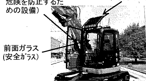
運転室周りの飛来物防護設備の例
